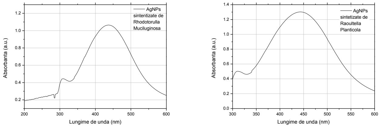
Fig. 5.3 Spectrele UV-vizibil ale coloizilor cu nanoparticule AgCl, biosintetizate de Rhodotorula Muciluginosa , respectiv Raoultella Planticola
